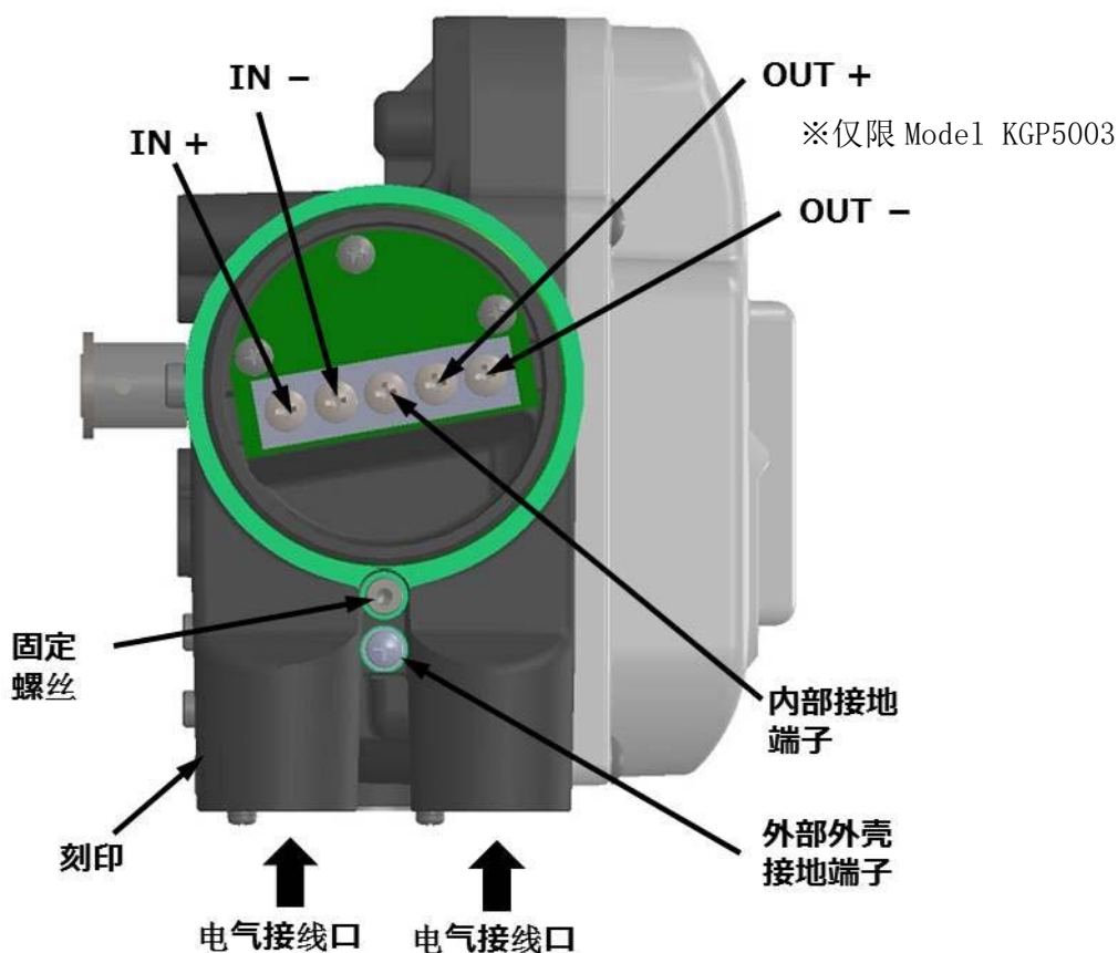
图 2.6a 电气接线口和端子
