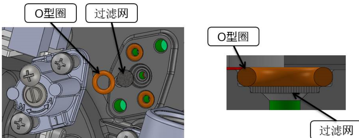
图 5.4.2 过滤部
