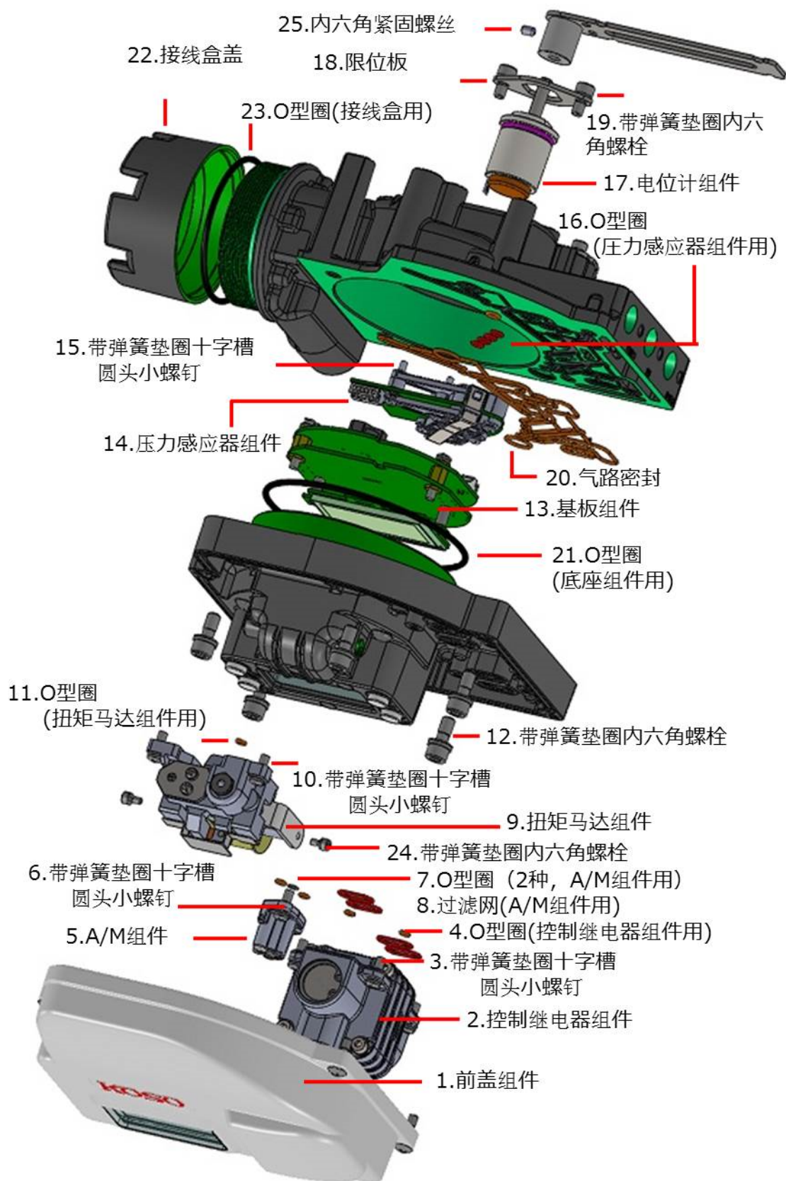
图 10.1 KGP5000 分解图和零件编号
