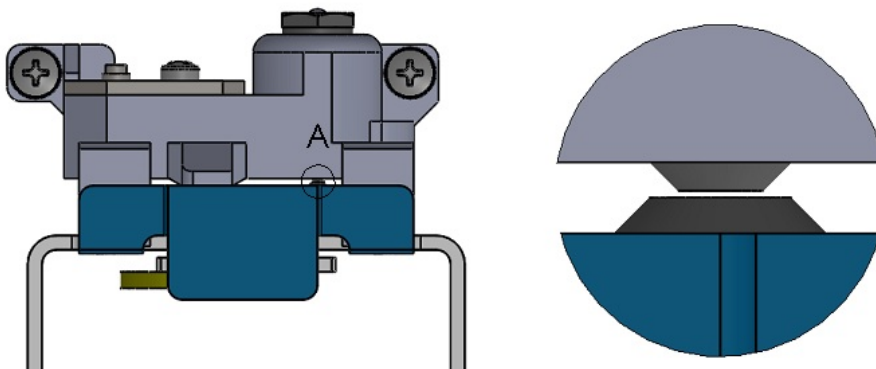
图 5.4.3 喷嘴挡板部
