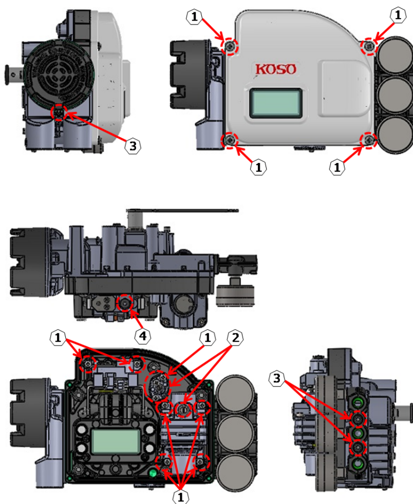
图 1.7 工具的使用部位
