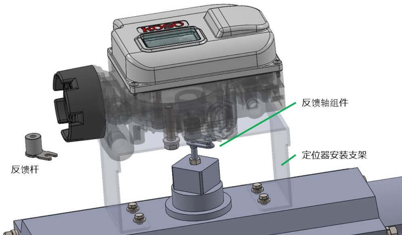
图 2.3 角行程执行机构安装示例
