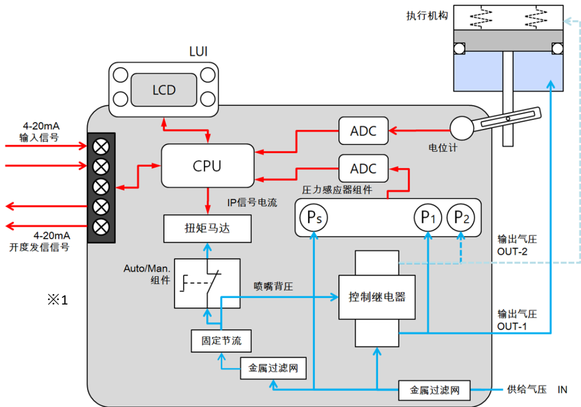
图 1.3.2a 模块构成
