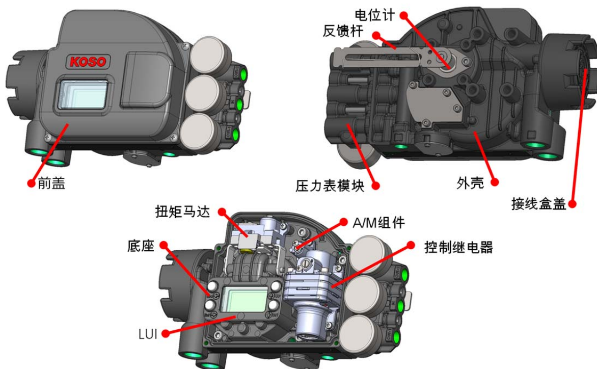
图 1.3.1 此装置的构成
