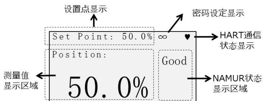
图 4.1.3b 监视画面的说明
