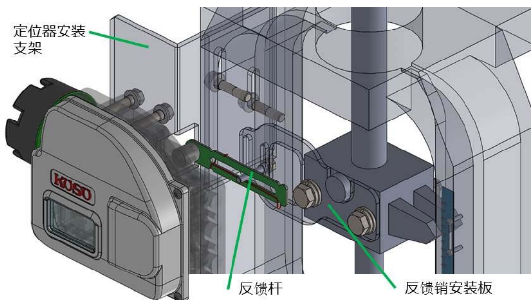
图 2. 2a 直行程执行机构安装示例
