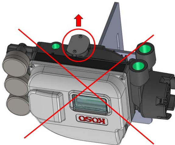
图 2.1a 颠倒上下的错误安装示例 (N.G. 例)
