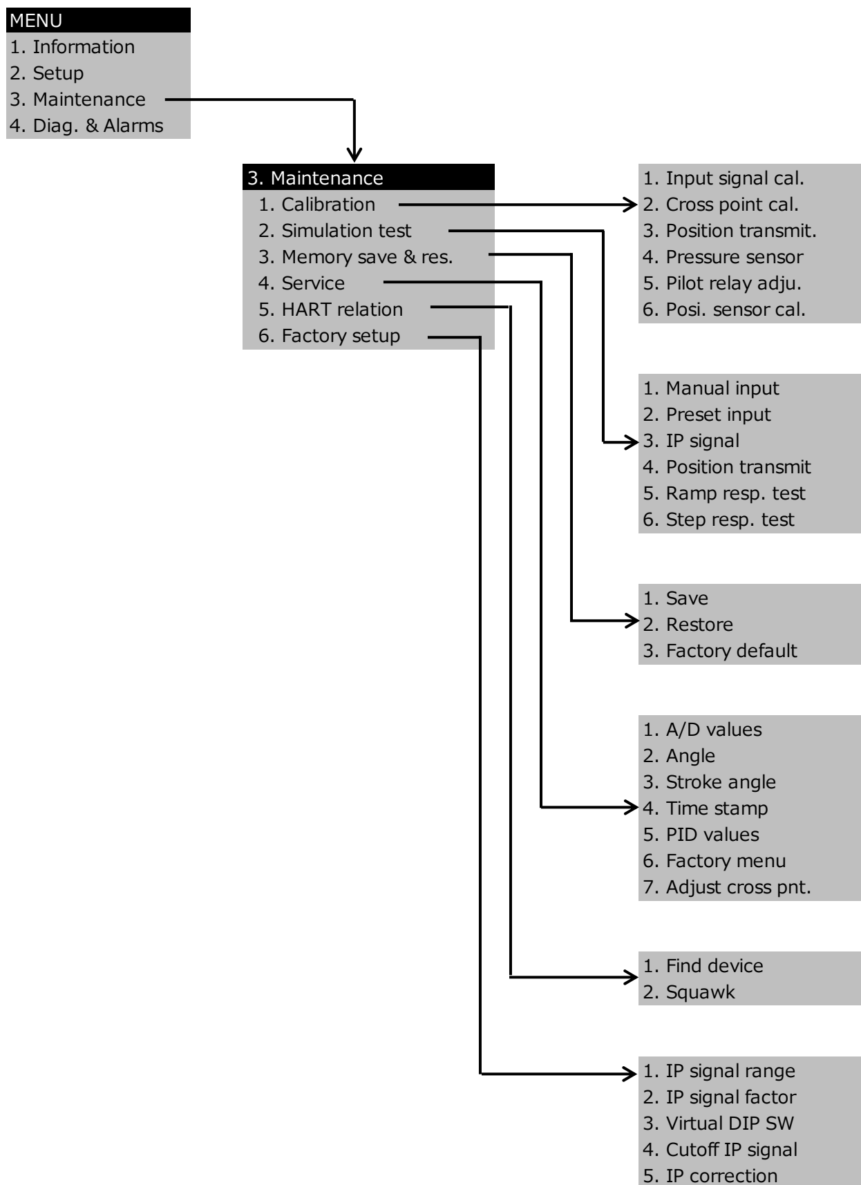
图 4. 1. 4c 维护保养菜单
