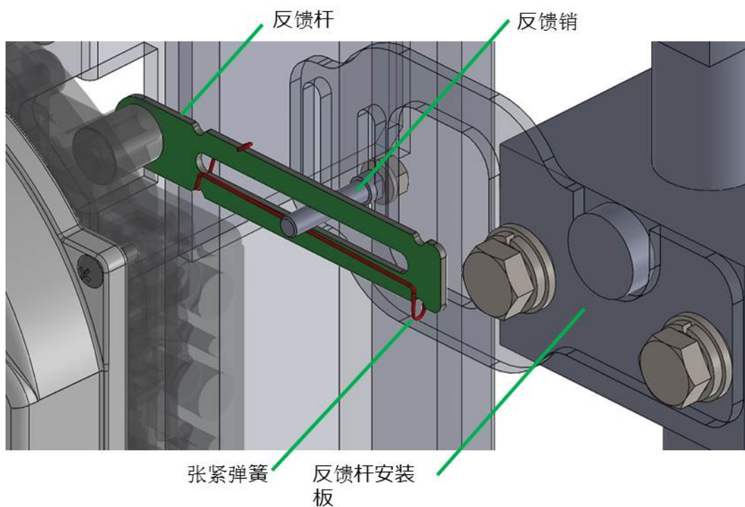
图 2.2b 张紧弹簧安装位置
