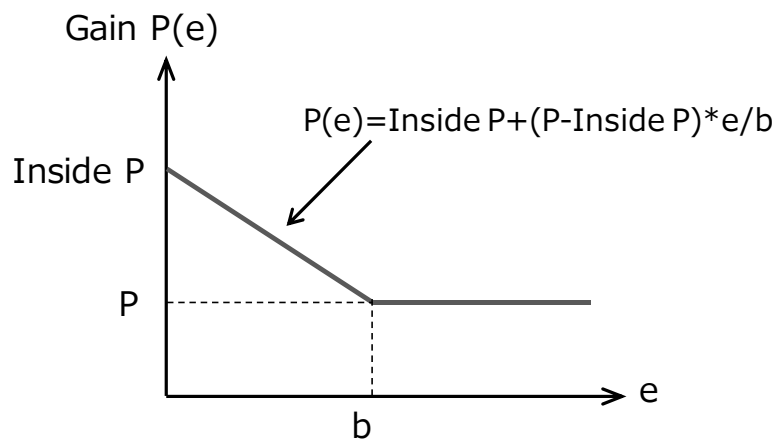
图 4.5.2. 增益切换 （以比例增益为例）
