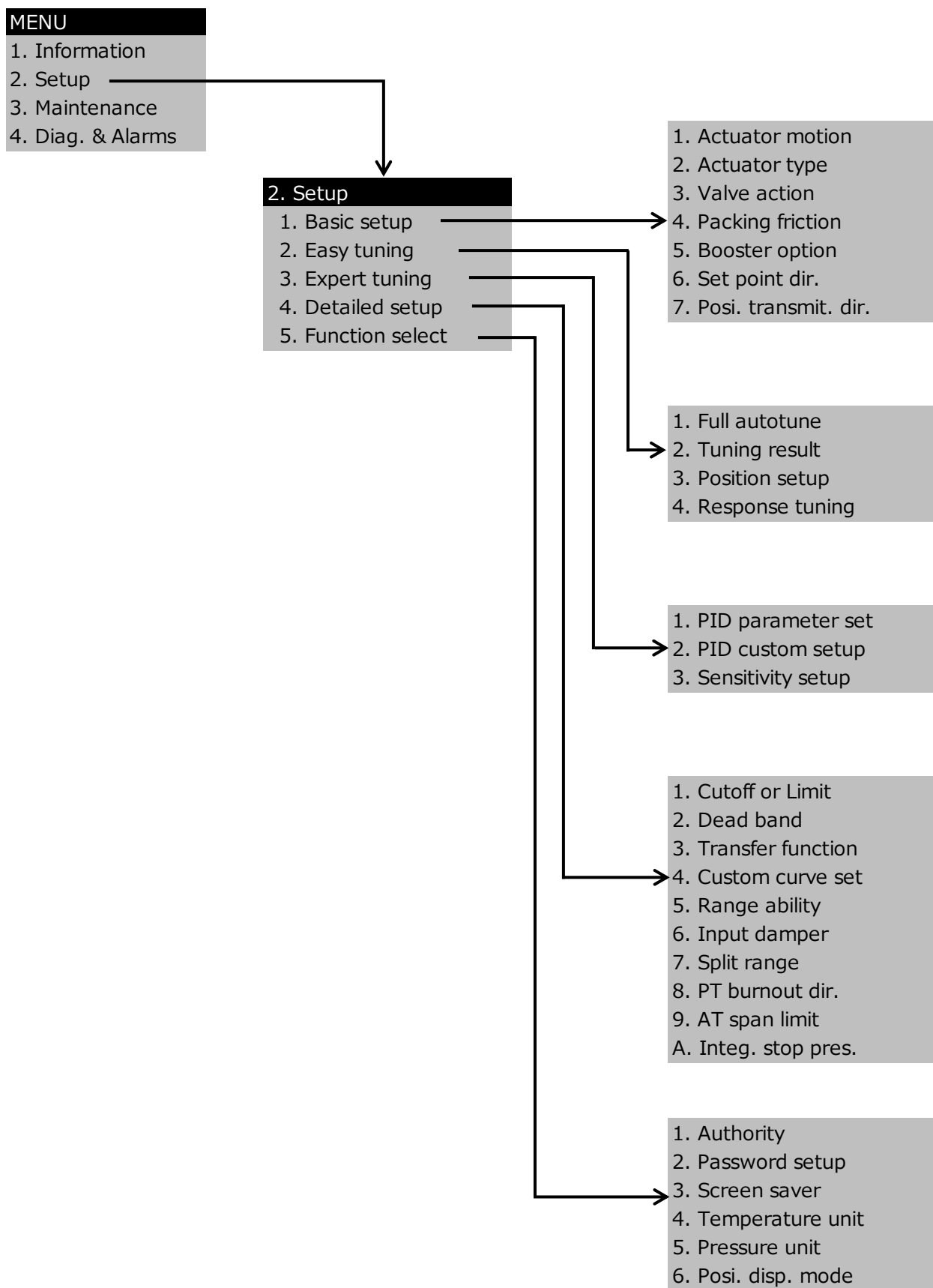
图 4. 1. 4b 设定菜单
