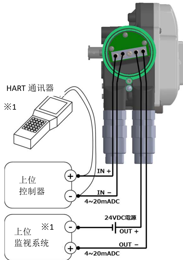
图 2.6e 电缆 2 根 (2 芯) 接线配线
