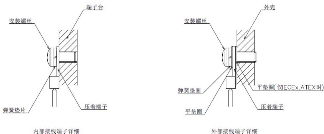
图 2.6c 接线端子详细图
