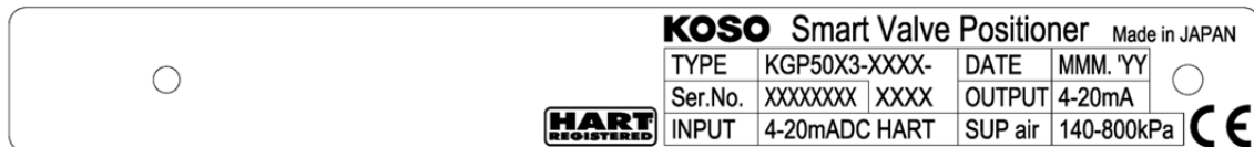
图. 1.5.1 标牌例 (非防爆型)
