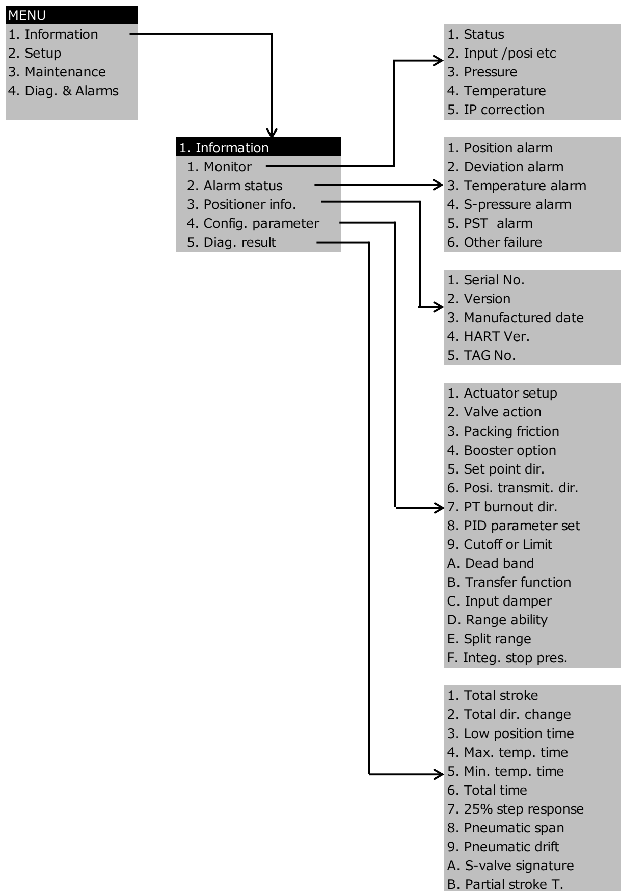
图 4.1.4a 信息菜单
