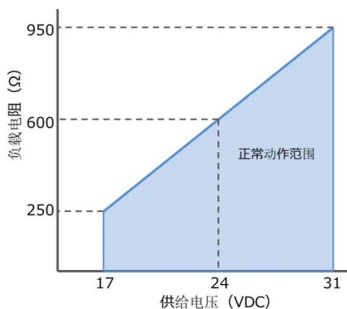
图 2.6f 开度发信接线时负载电阻和供压关系图
