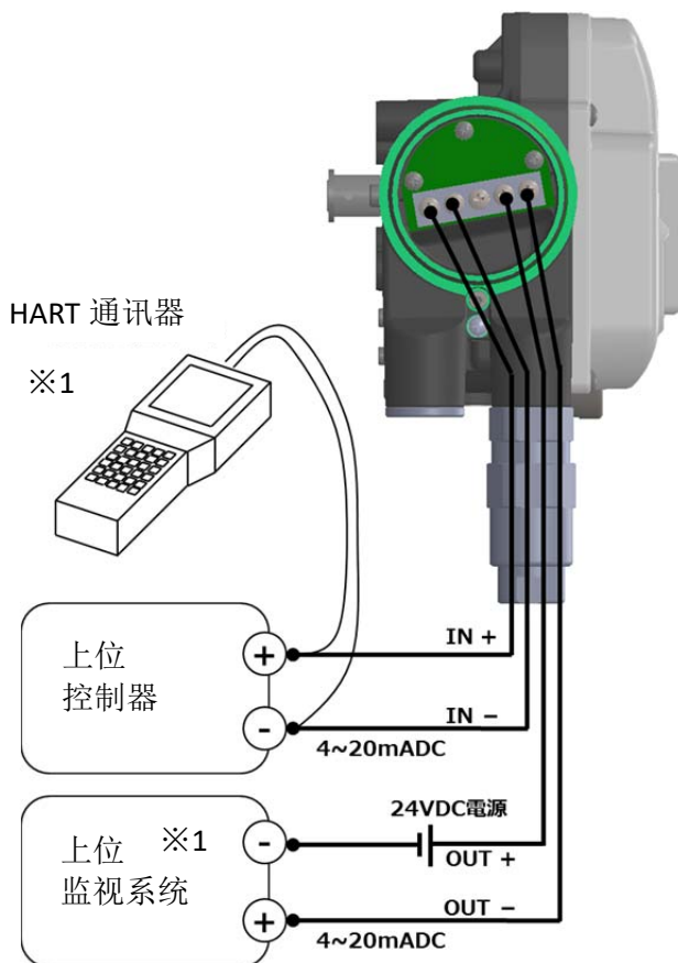
图 2.6d 电缆 1 根 (4 芯) 接线配线
