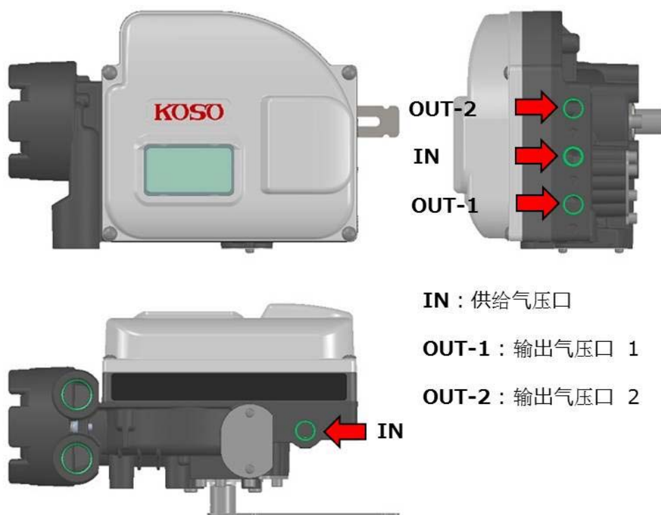
图 2.5 空气接口
