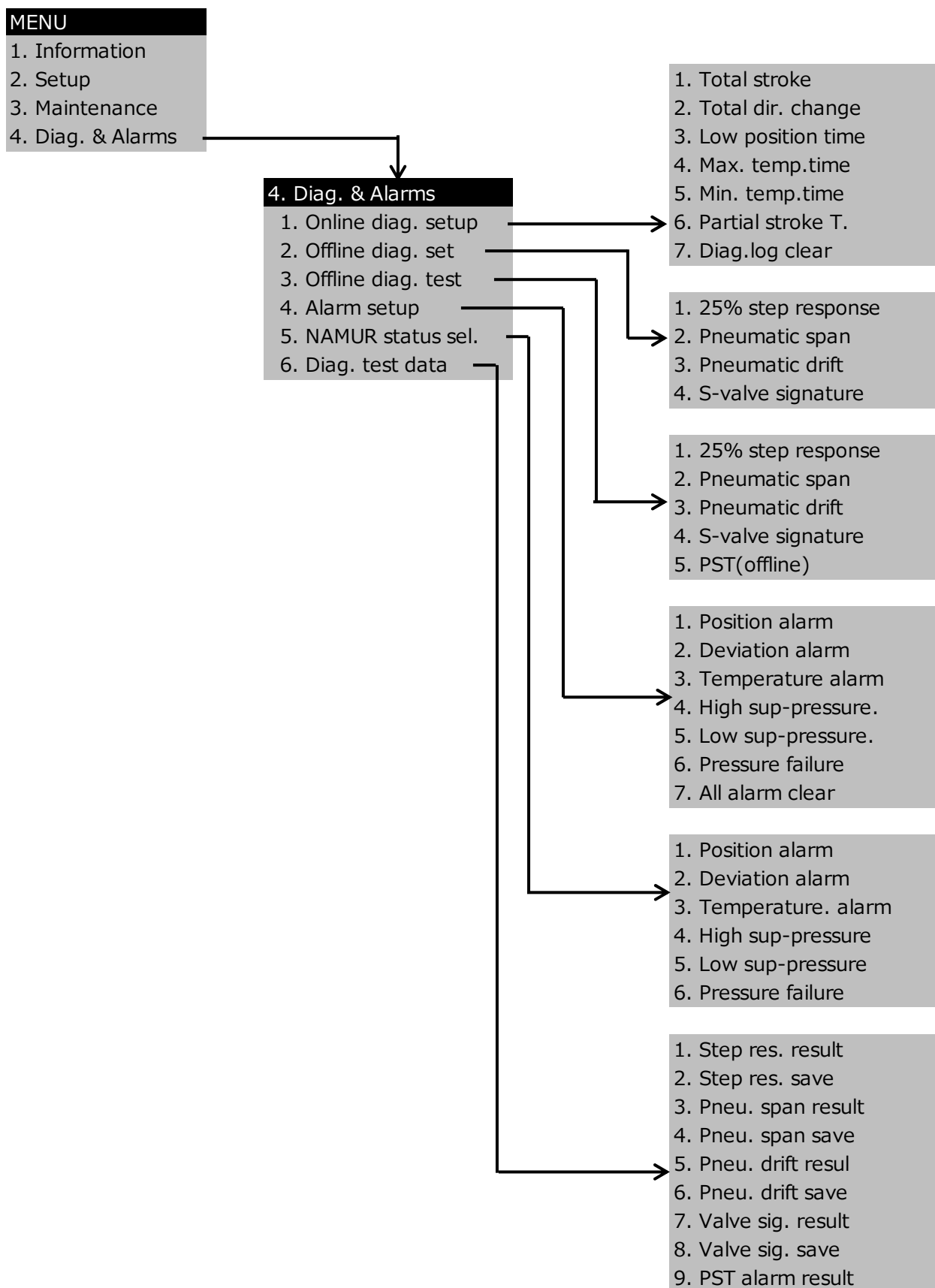
图 4. 1. 4d 诊断&警报菜单
