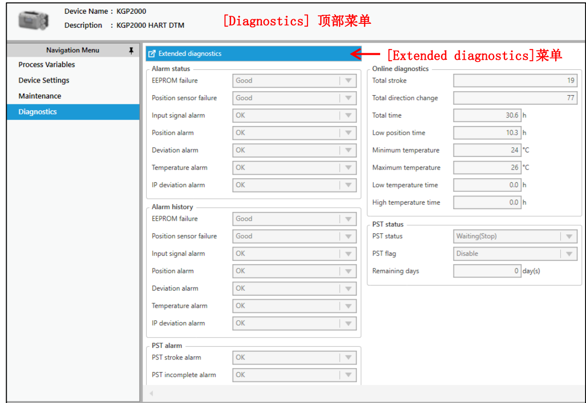
图 2.2.4a [Diagnostics]顶部菜单
