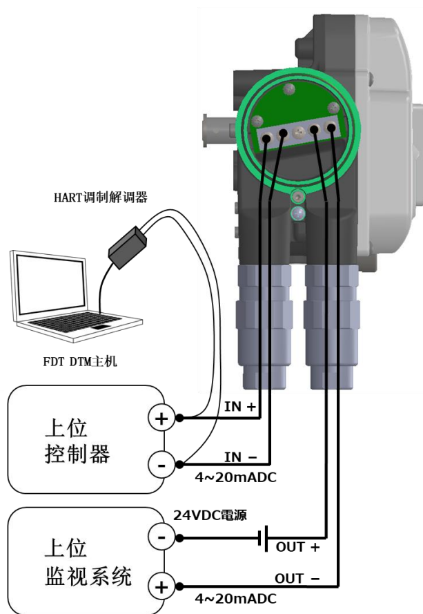
图 1.4c 电缆 2 根 (2 芯) 接线配线
