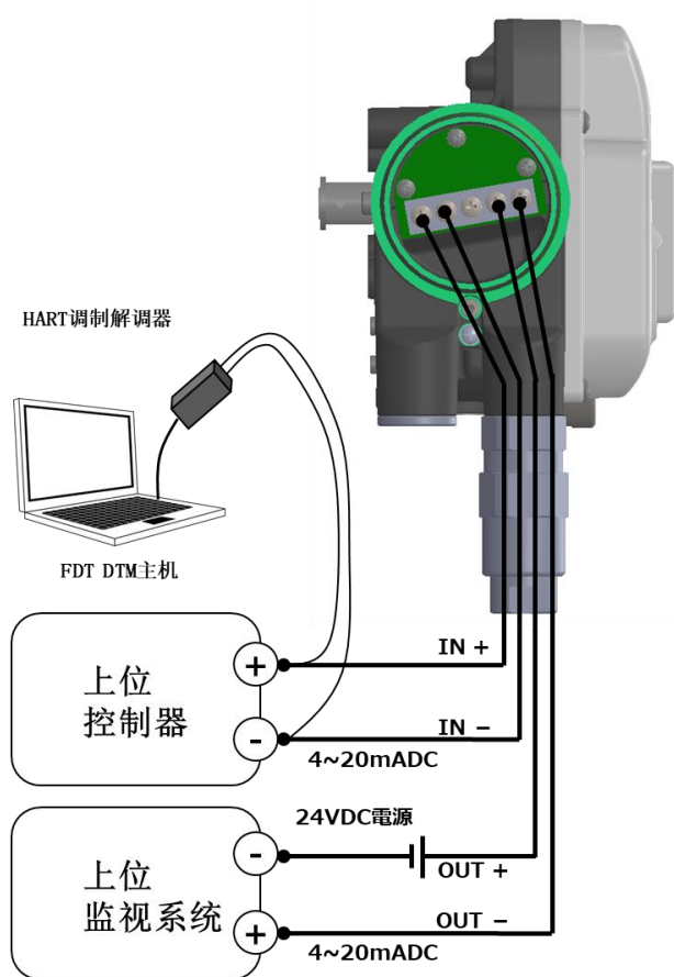
图 1.4b 电缆 1 根 (4 芯) 接线配线
