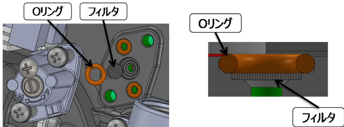
図 5.4.2 フィルタ部
