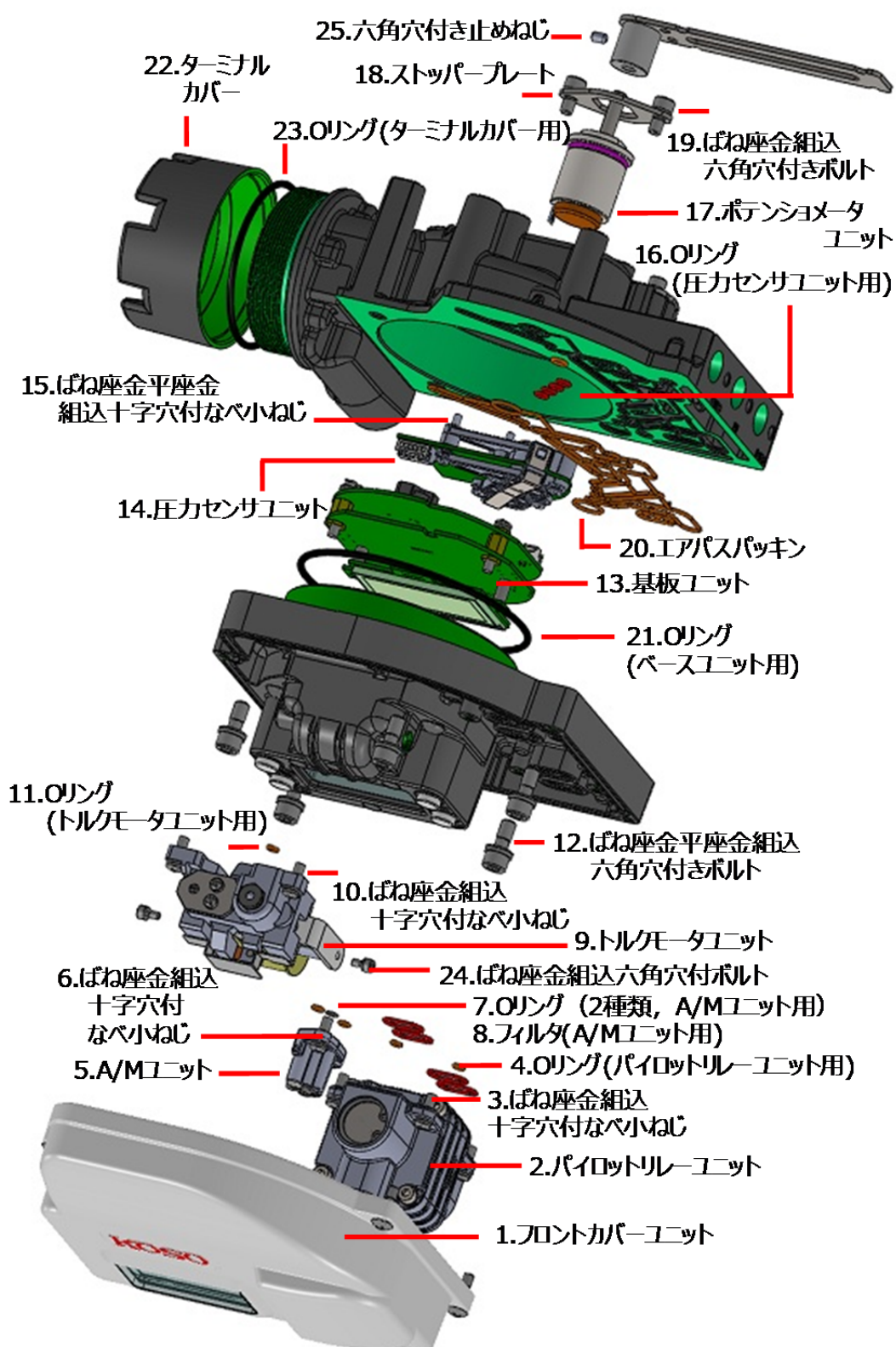
図 10.1 KGP5000 分解図と部品番号
