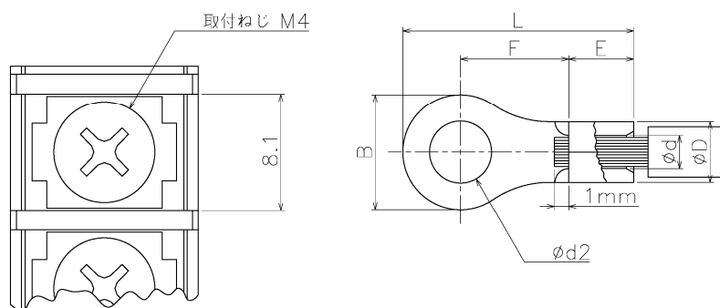
図 2.6b 圧着端子の例
