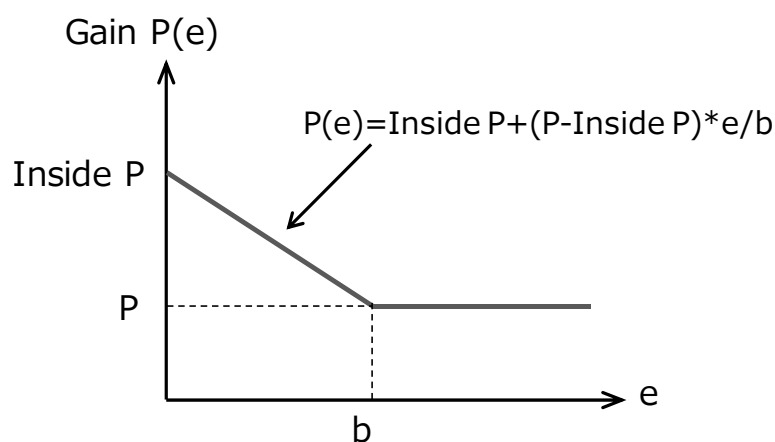
図 4.5.2. ゲイン切り替え（例. 比例ゲインの場合）
