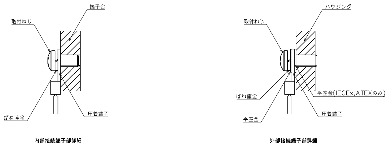
図 2.6c 接続端子部詳細
