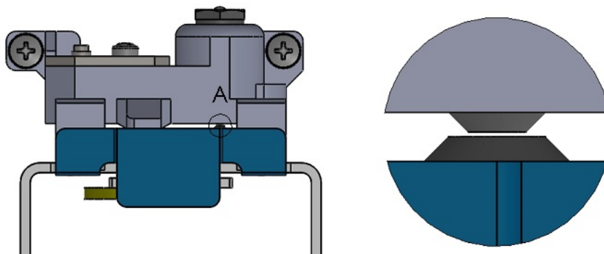
図 5.4.3 ノズルフラップ部
