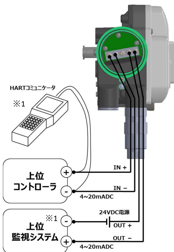
図 2.6d ケーブル 1 本(4 芯)による電気配線
