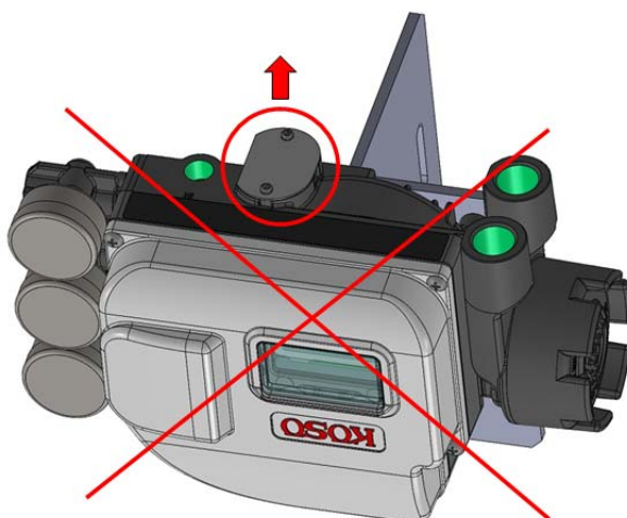
図 2.1a 天地逆取り付けの例 (N.G.例)
