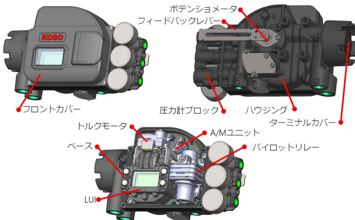
図 1.3.1 本器の構成
