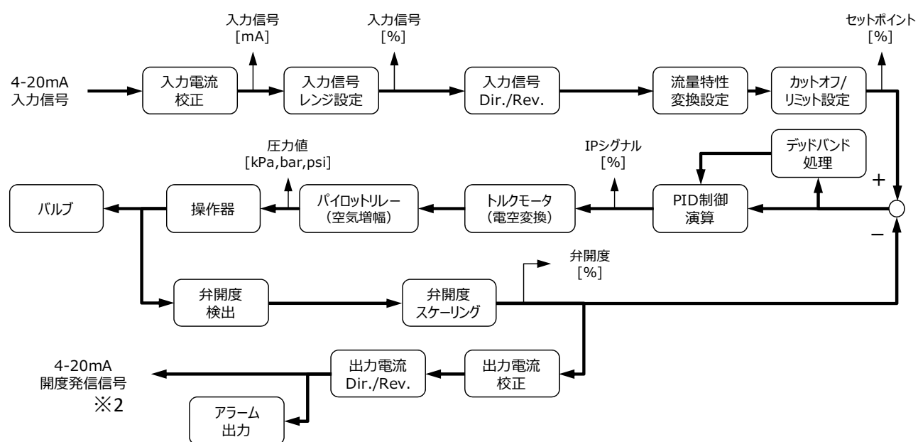
図 1.3.2b 入出力処理フロー
