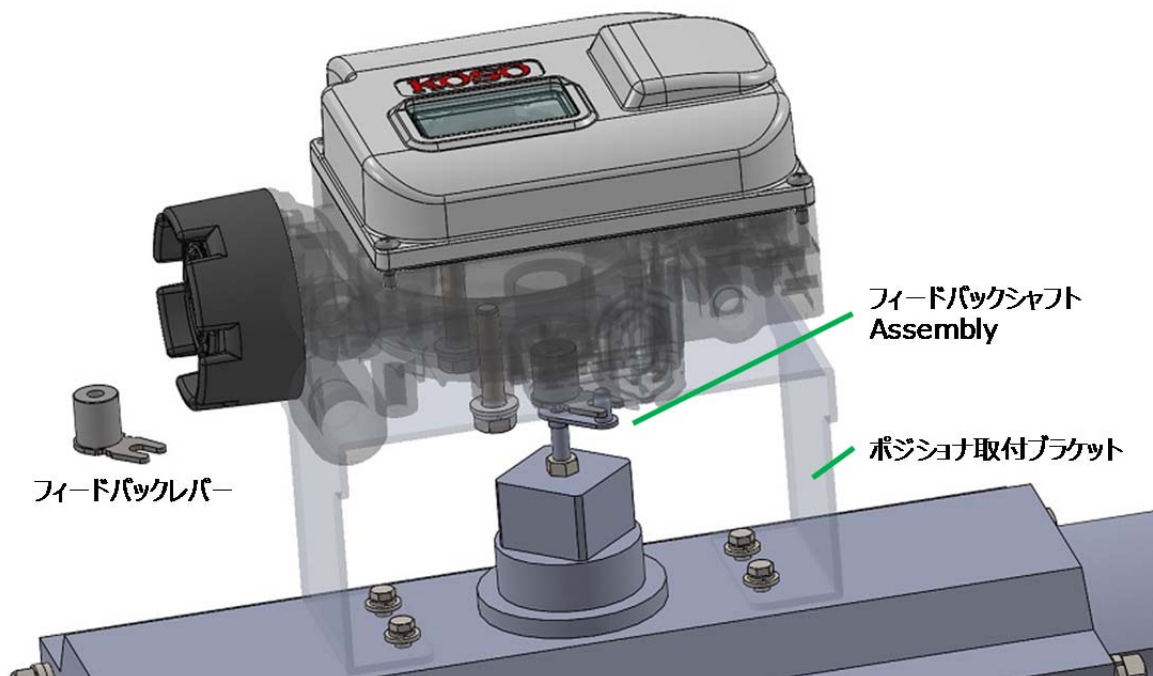
図 2.3 回転運動形駆動部への取り付け例
