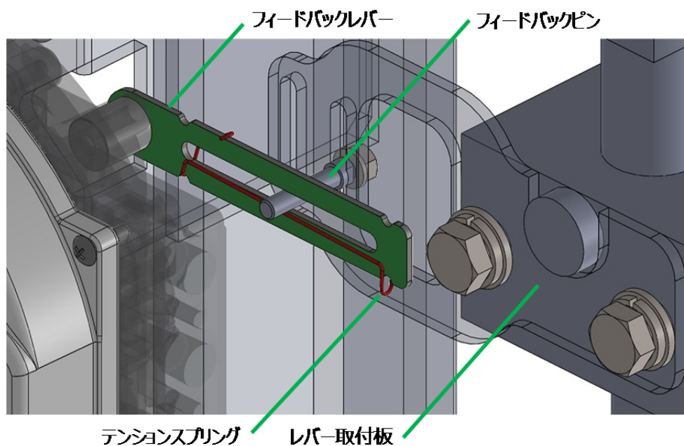
図 2.2b テンションスプリングの組付位置
