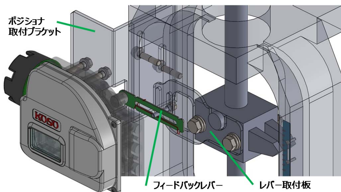
図 2.2a 直線運動形駆動部への取り付け例
