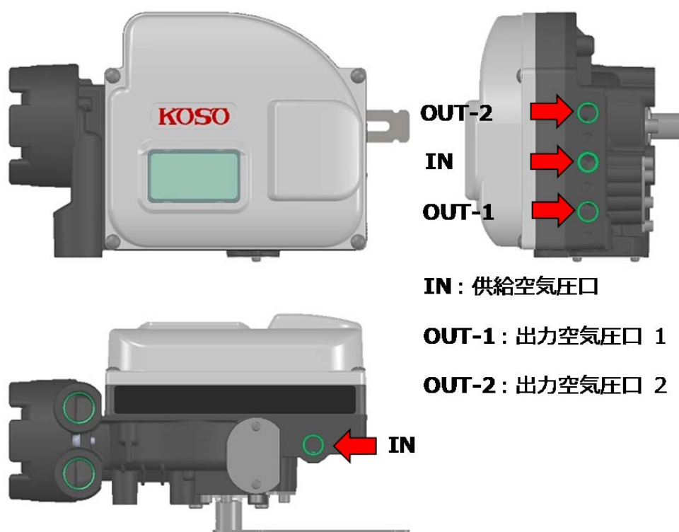
図 2.5 空気接続口
