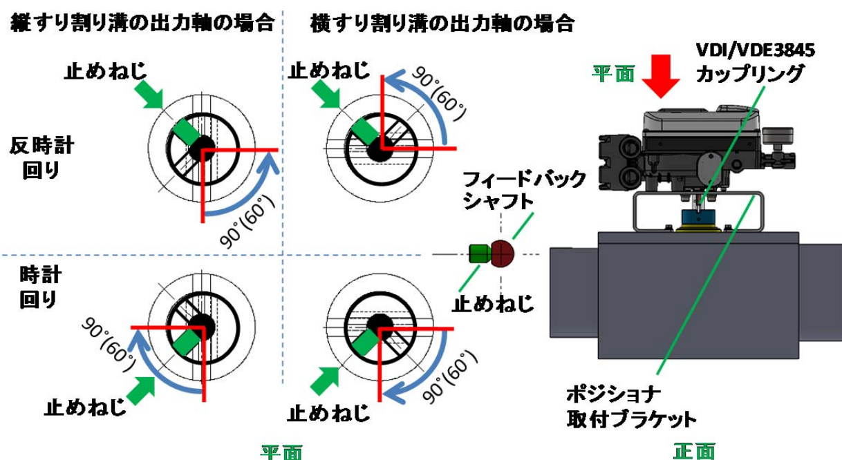
図 2.4 回転運動形駆動部への取り付け例
