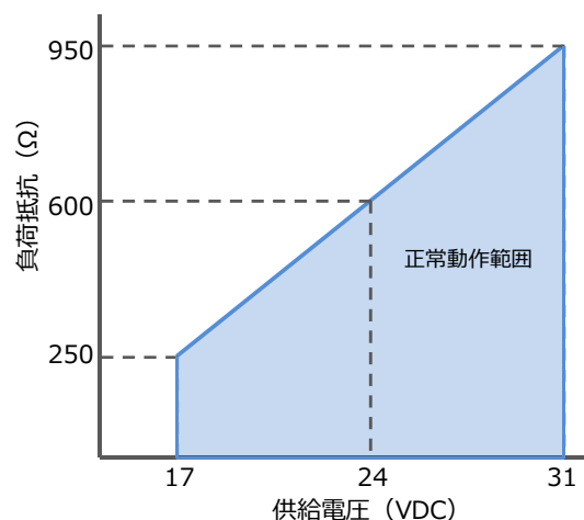
図 2.6f 開度発信接続における負荷抵抗と供給電源電圧
