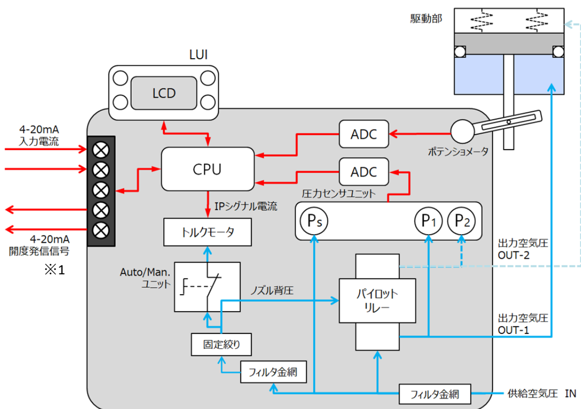
図 1.3.2a ブロック構成
