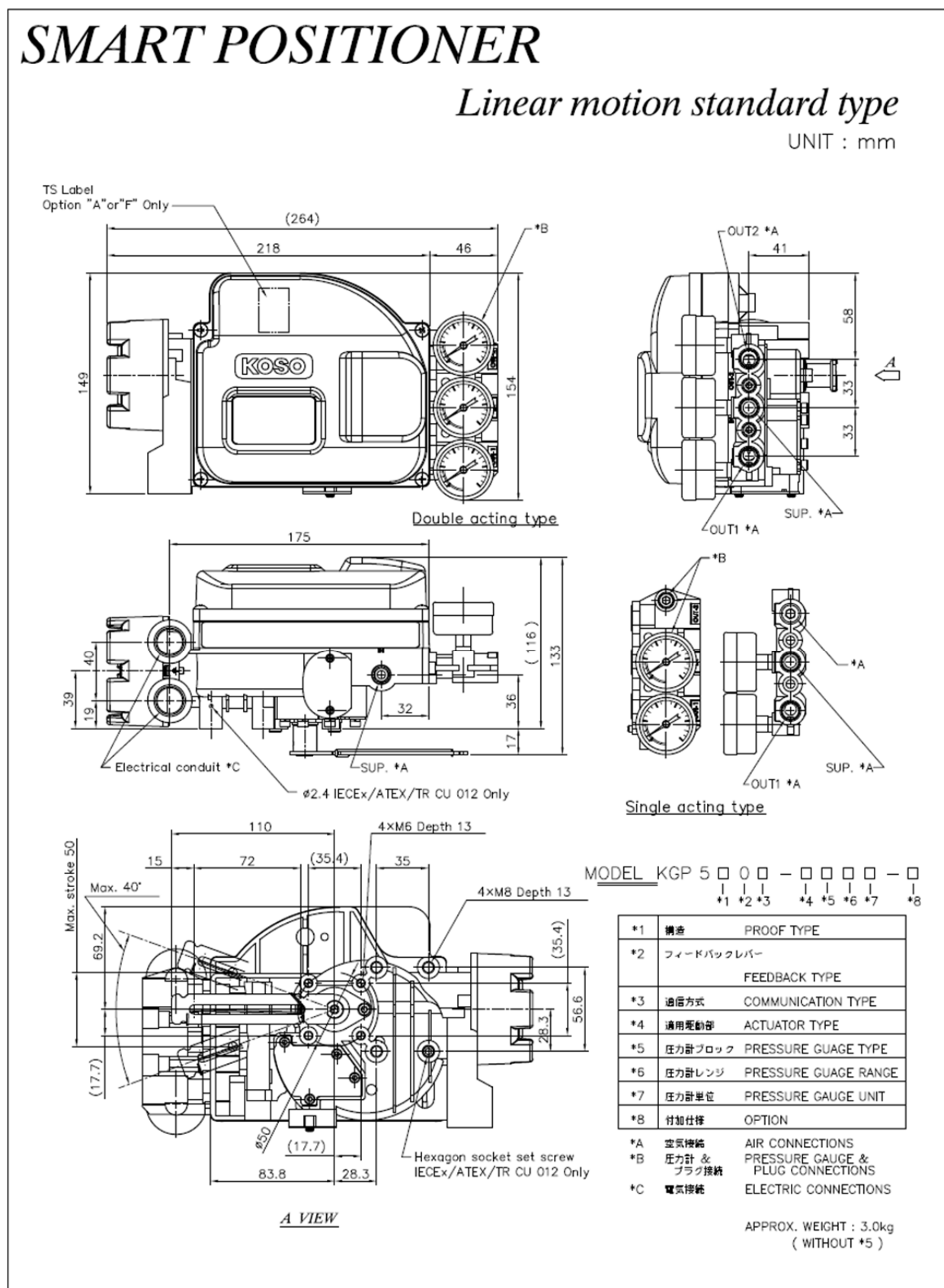
図 11a リニア用標準レバー形
