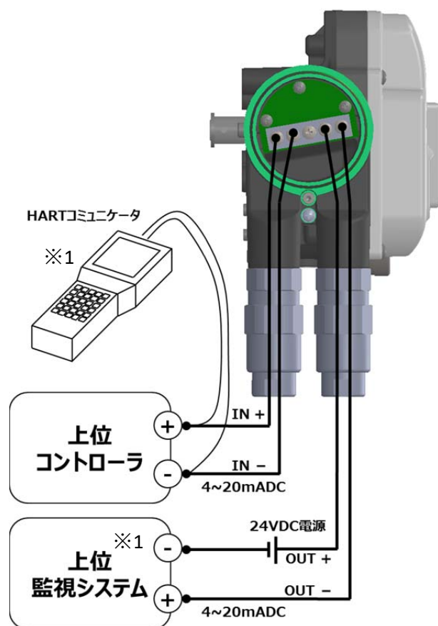
図 2.6e ケーブル 2 本(2 芯)による電気配線
